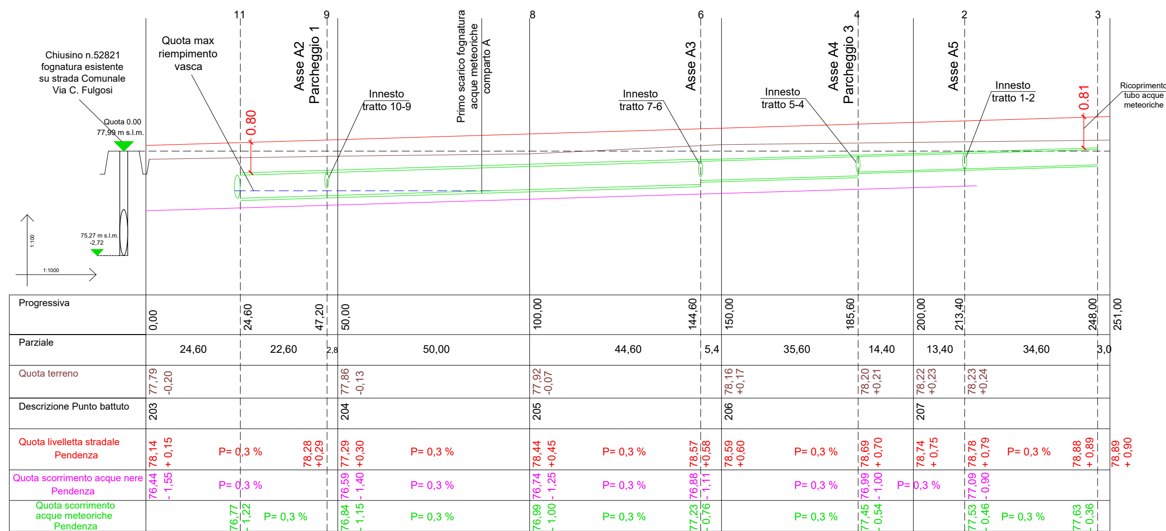
Sezione longitudinale lungo l'asse A1
