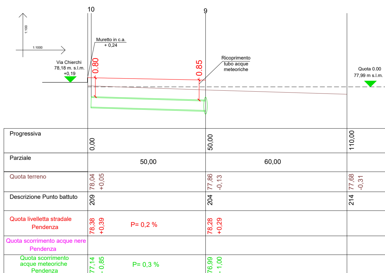
Sezione longitudinale lungo l'asse A2 Parcheggio 1
