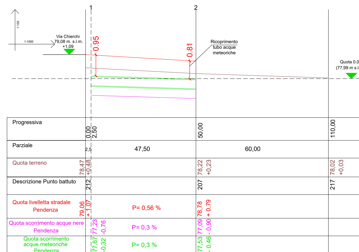
Sezione longitudinale lungo l'asse A5
