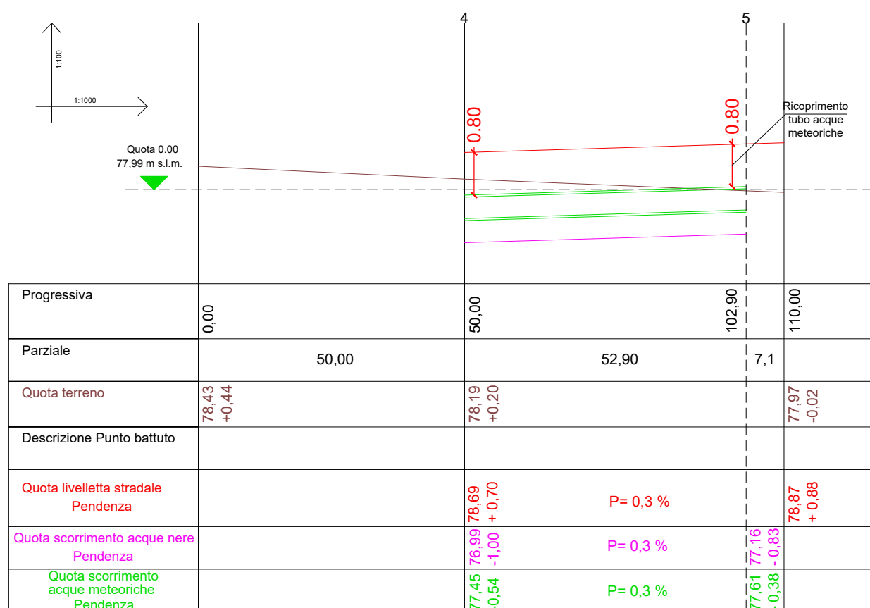
Sezione longitudinale lungo l'asse A4 Parcheggio 3
