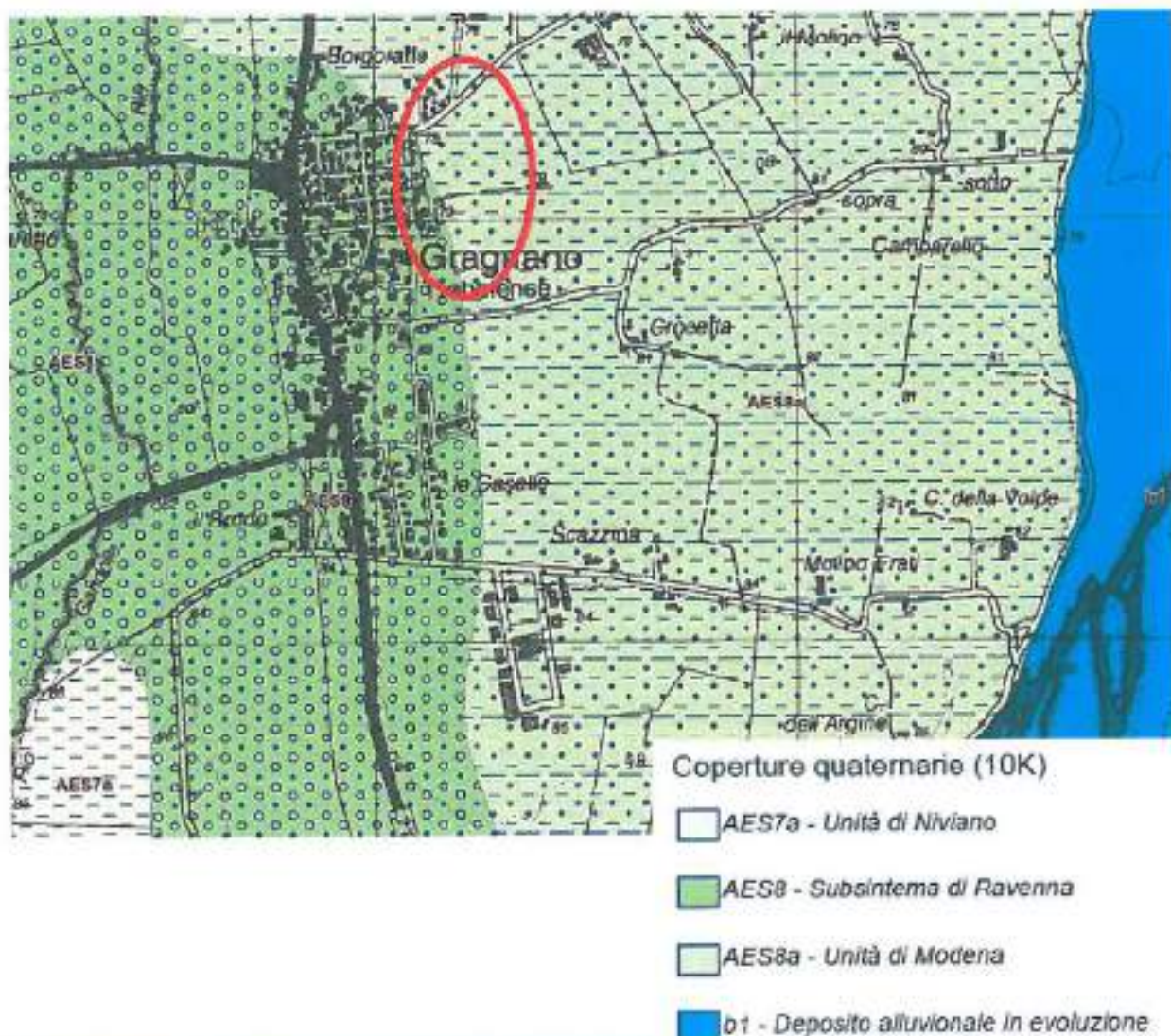
Fig. n. 3 carta geologica
