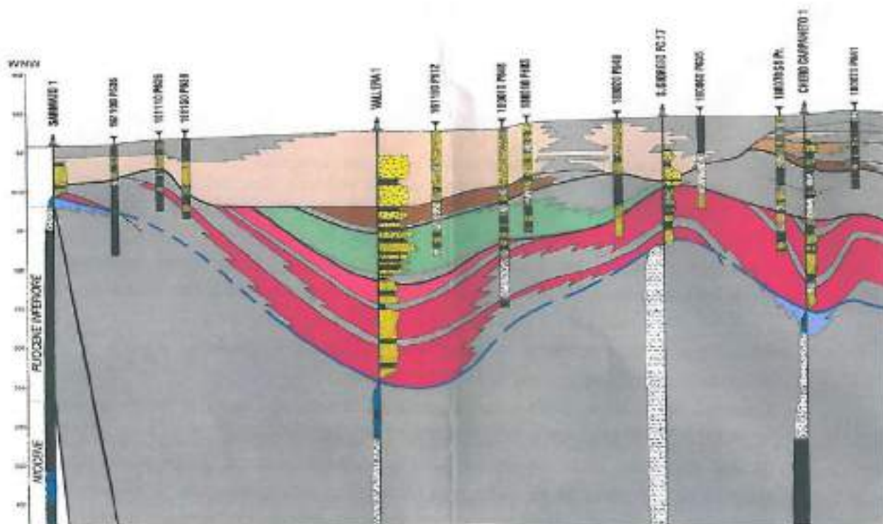
Sezione B ovest
