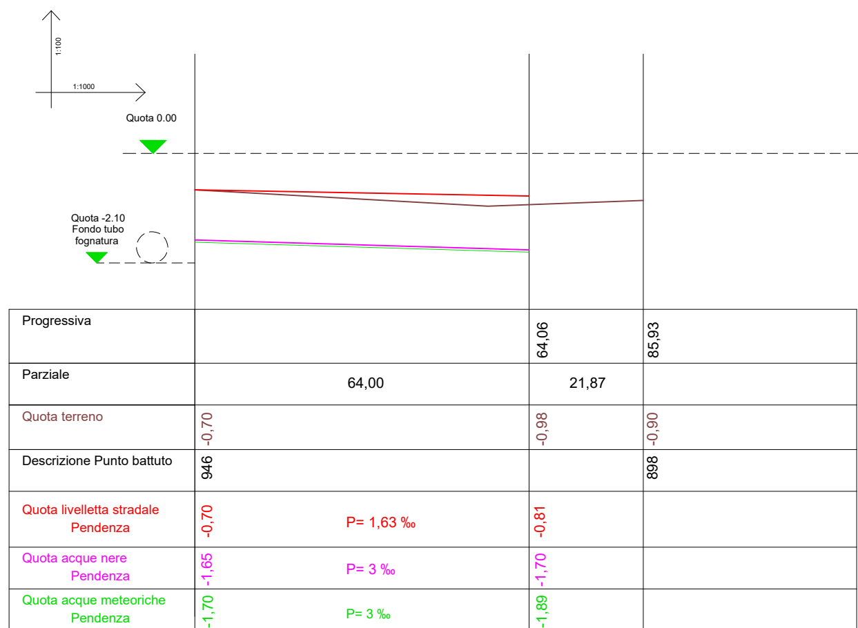
Sezione longitudinale lungo l'asse A3
