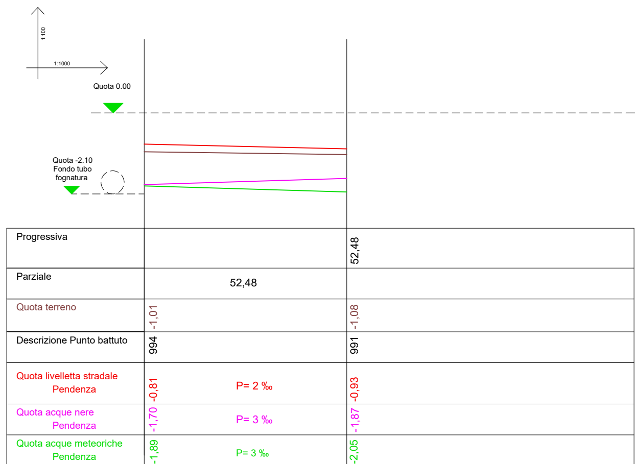
Sezione longitudinale lungo l'asse A2
