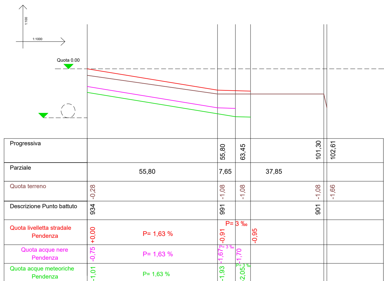
Sezione longitudinale lungo l'asse A1
