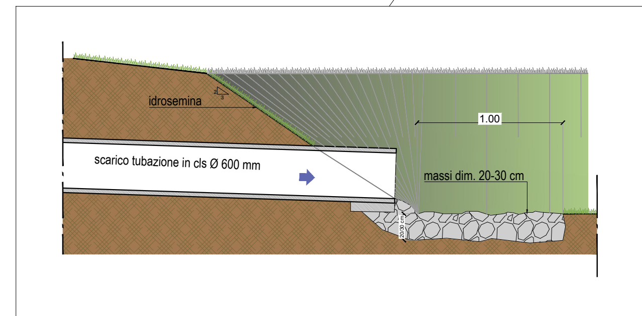
Particolare scarico in vasca (Scala 1:50)
