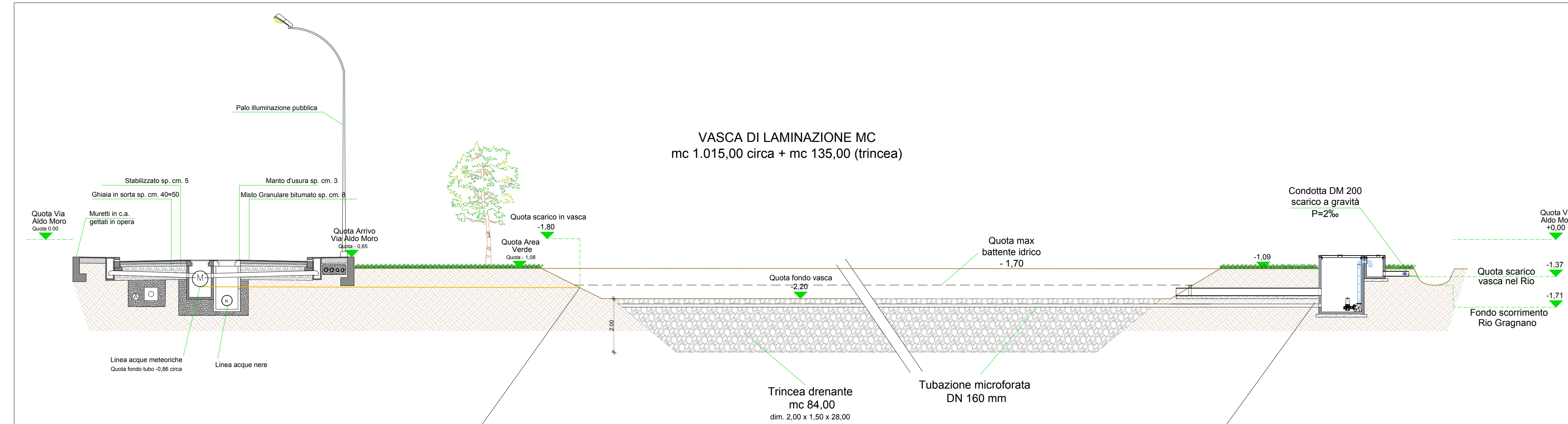
Sezione vasca (Scala 1:100)
