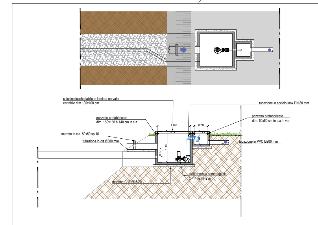
Particolare pozzetti scarico (Scala 1:100)
